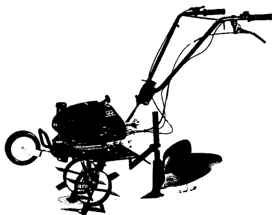
Häufelausrüstung
